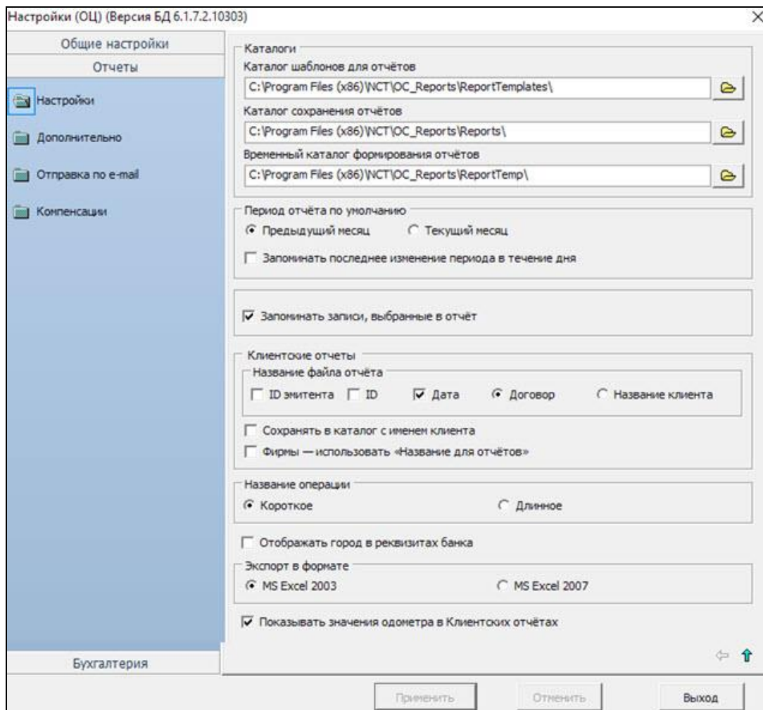
Рис. 9. Окно «Настройки»
