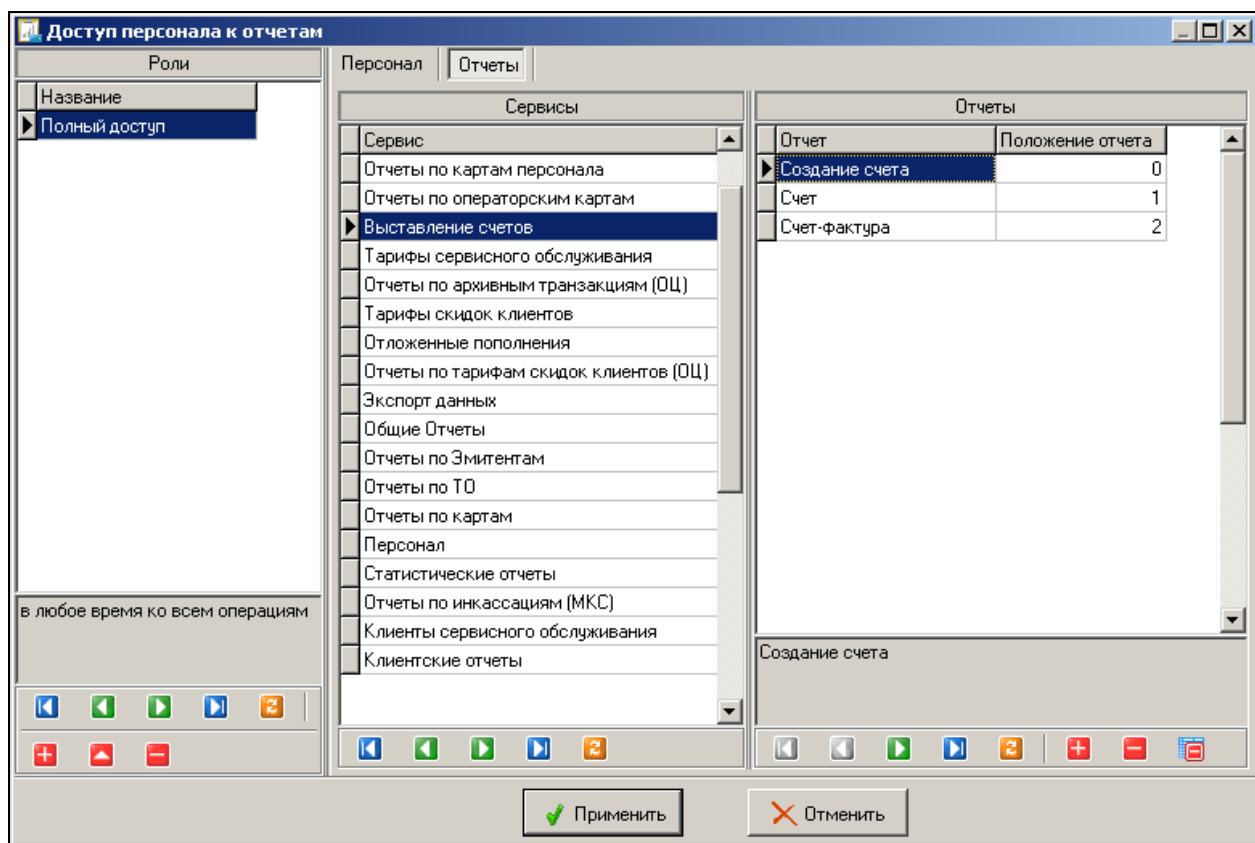
Рис. 6. Закладка «Отчеты»
