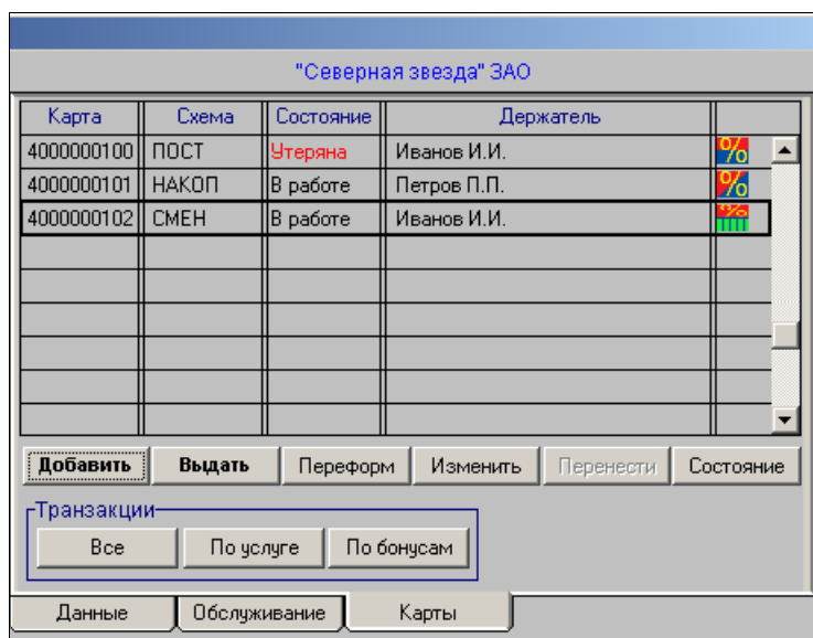
Рис. 38. Закладка «Карты»
