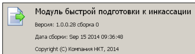
Рис. 16. О программе
