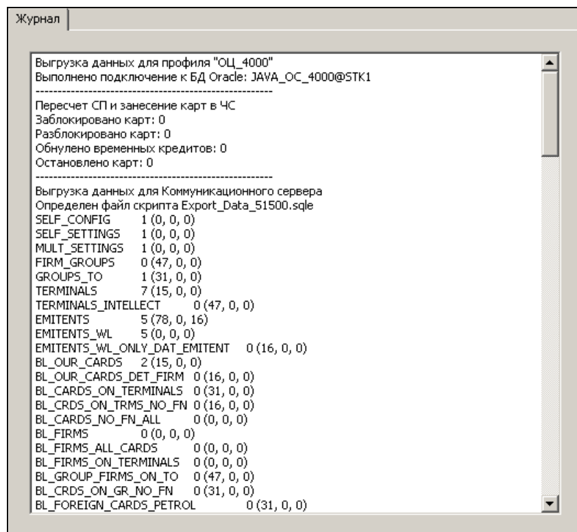
Рис. 15. Журнал выполнения
