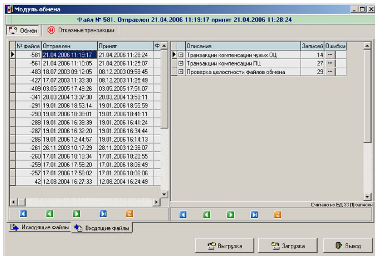
Рис. 64. Действия с входящими файлами
