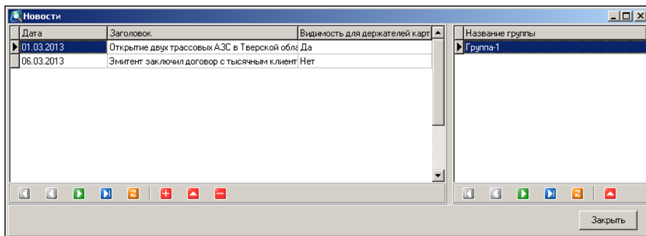
Рис. 97. Окно «Новости»
