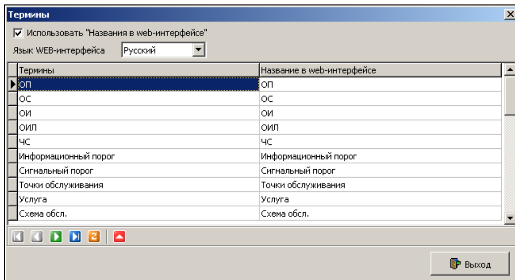
Рис. 94. Окно «Термины»
