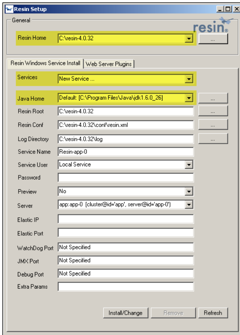
Рис. 23. Resin. Параметры установки службы веб-сервера
