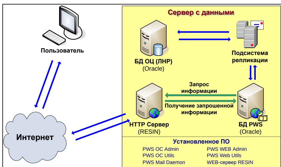
Рис. 4. Схема установки компонентов №4 (все компоненты на одном сервере)
