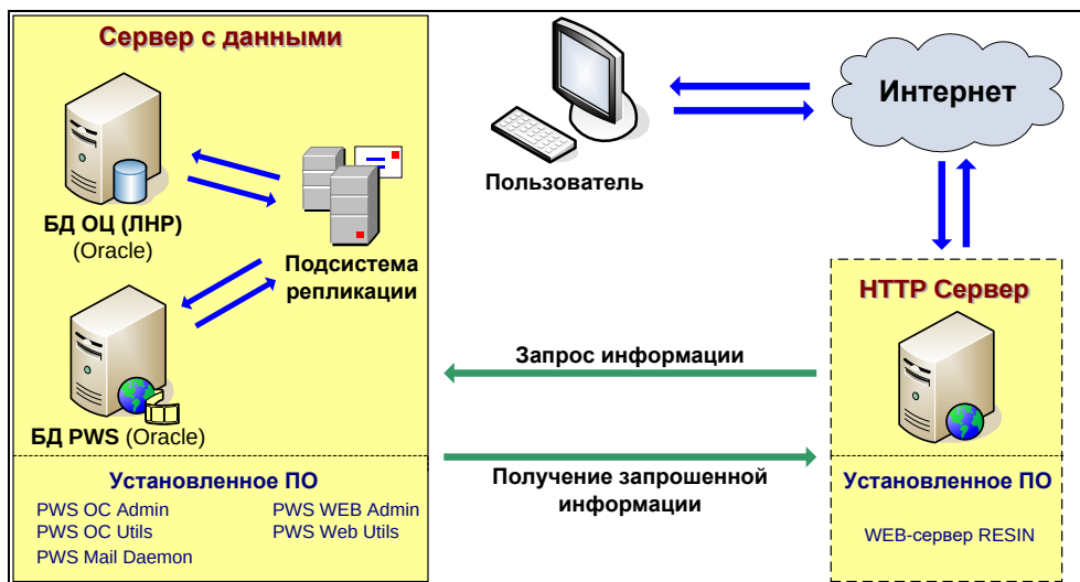
Рис. 3. Схема установки компонентов №3 (ОЦ и PWS на одном сервере)
