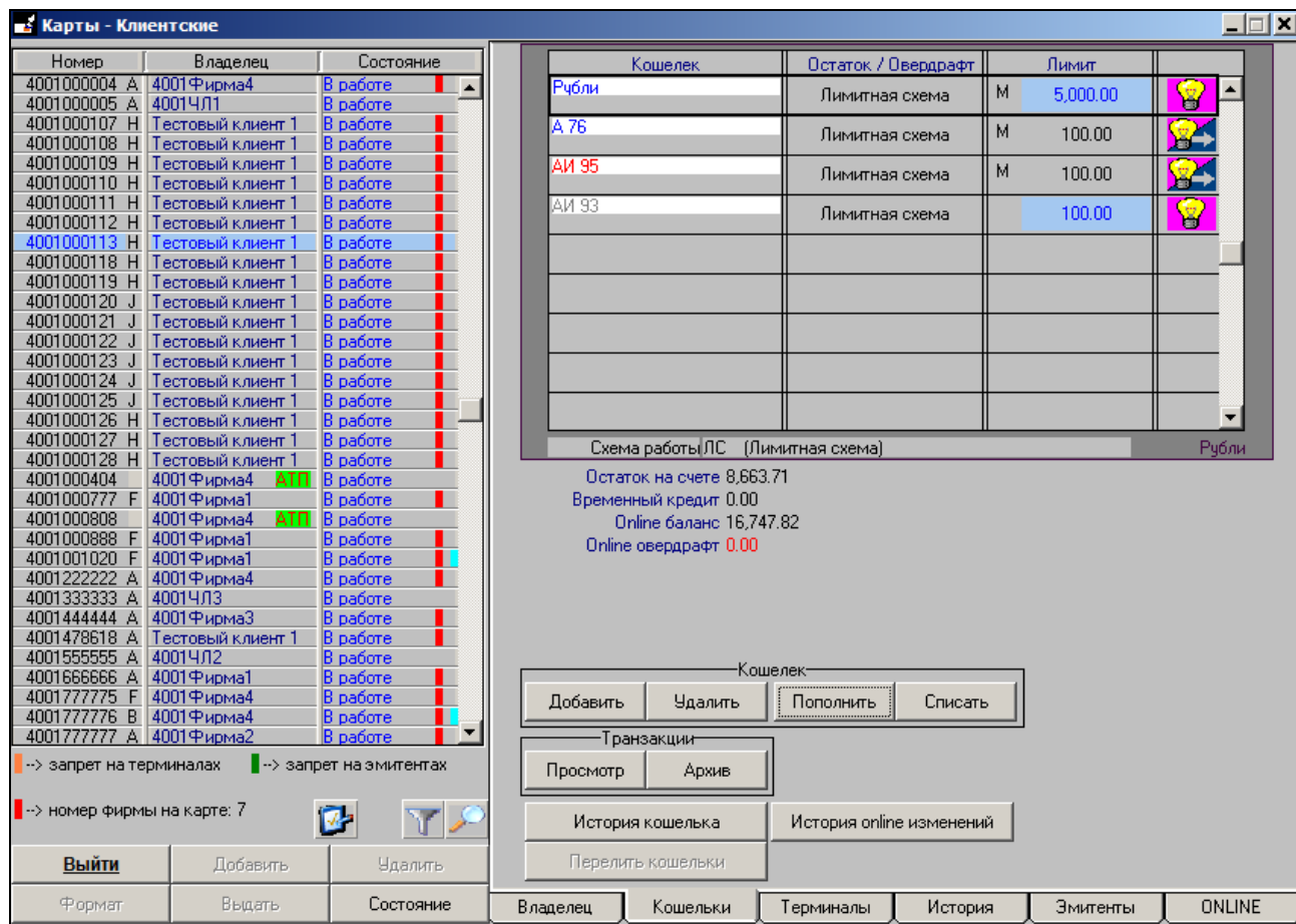
Рис. 45. Окно «Карты - Клиентские». Закладка «Кошельки»
