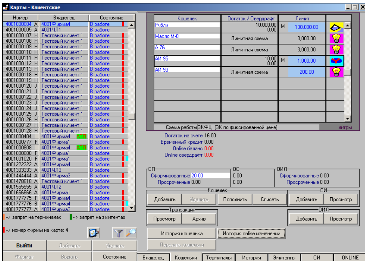
Рис. 1. Вид закладки «Кошельки» окна «Карты – Клиентские» при подключённых модулях «ONLINE», «ONLINE кошелек», «ОП», «ОС» и «ОИЛ»
