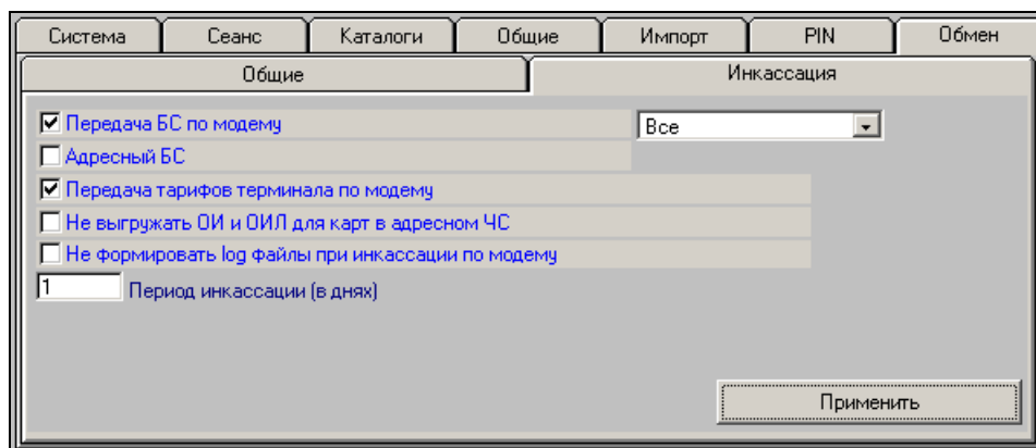
Рис. 1. Окно «Конфигурация системы». Закладка «Обмен / Инкассация»
