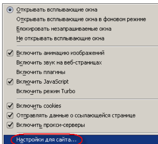
Рис. 20. Opera 12. Быстрые настройки. Пункт «Настройки для сайта...»
