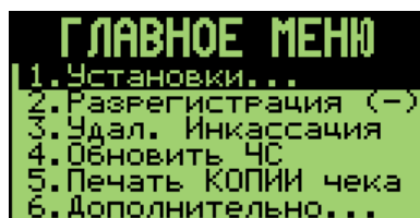
Рис. 1. «Главное меню»
