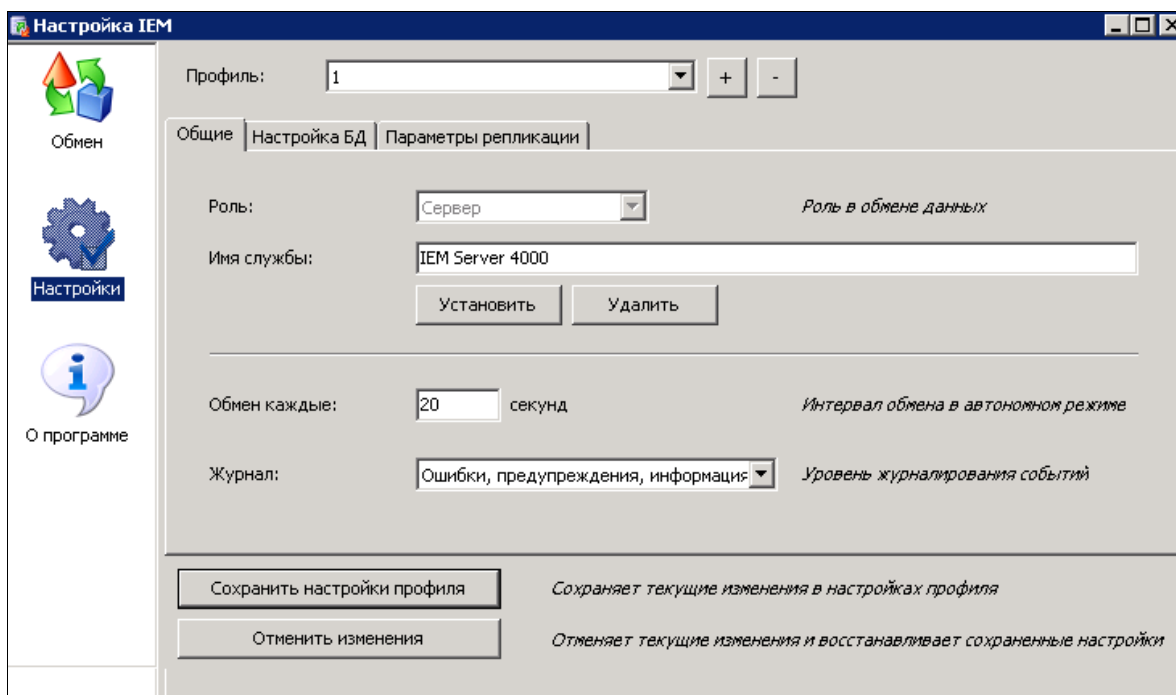
Рис. 14. Рабочая область настроек программы IEM-AS (сервер)
