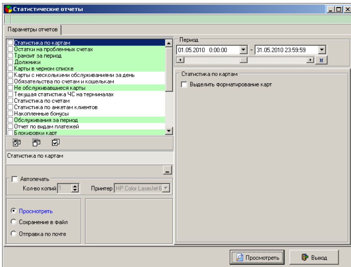
Рис. 1. Окно Сервиса
