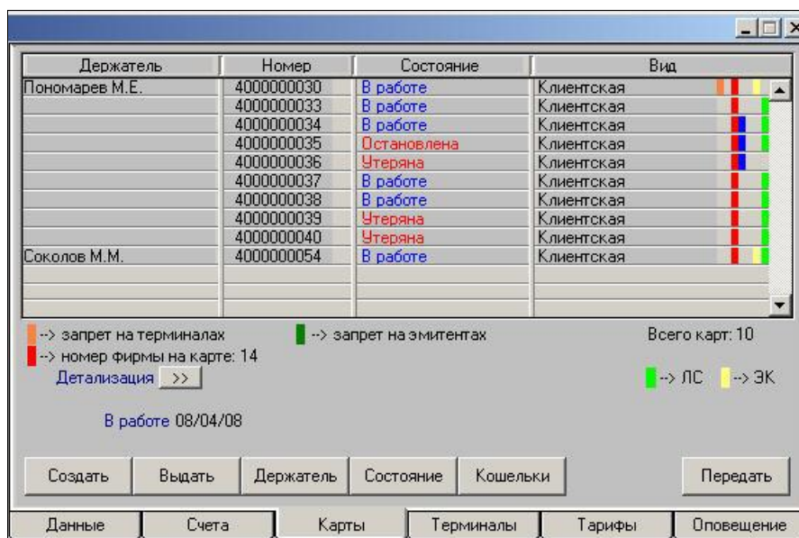
Рис. 19. Окно «Фирмы - В работе». Закладка «Карты»
