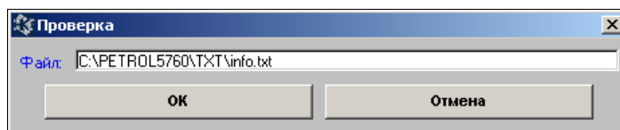
Рис. 30. Окно «Проверка»
