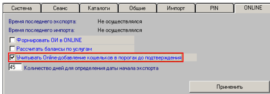
Рис. 8. Окно «Конфигурация системы». Закладка «ONLINE»
