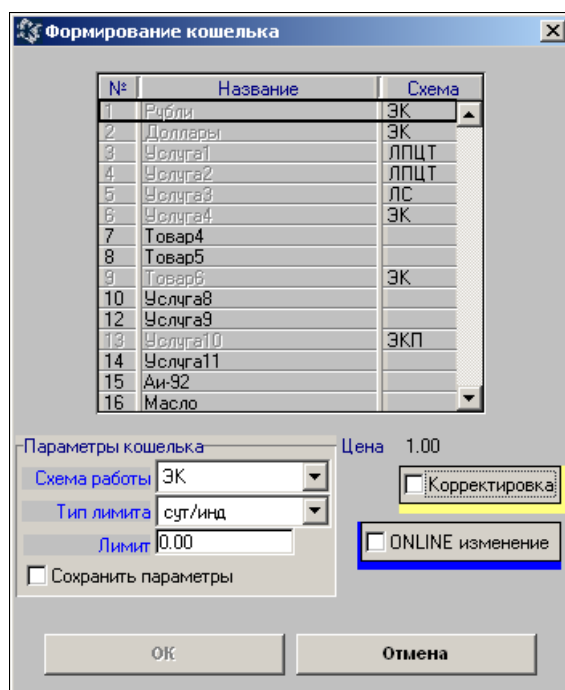
Рис. 3. Окно «Формирование кошелька»
