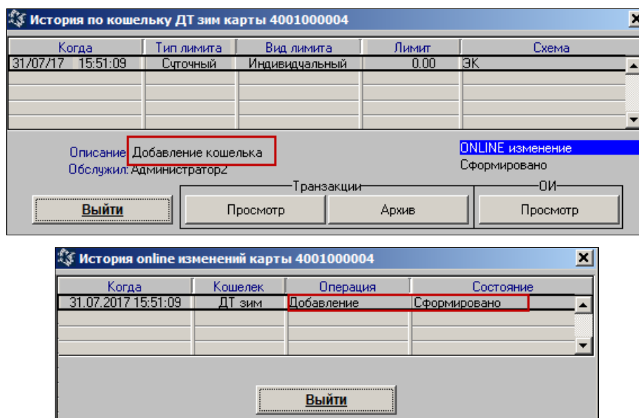
Рис. 5. Просмотр online-изменения на добавление кошелька
