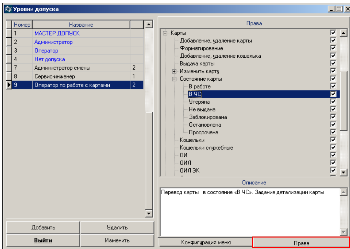
Рис. 1. Окно «Уровни допуска»
