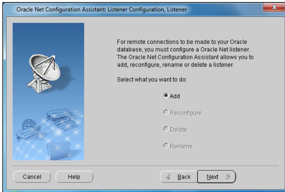
Рис. 40. Добавление Listener
