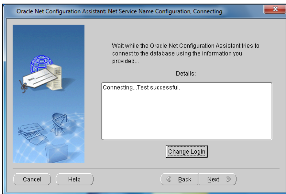
Рис. 52. Результат тестирования
